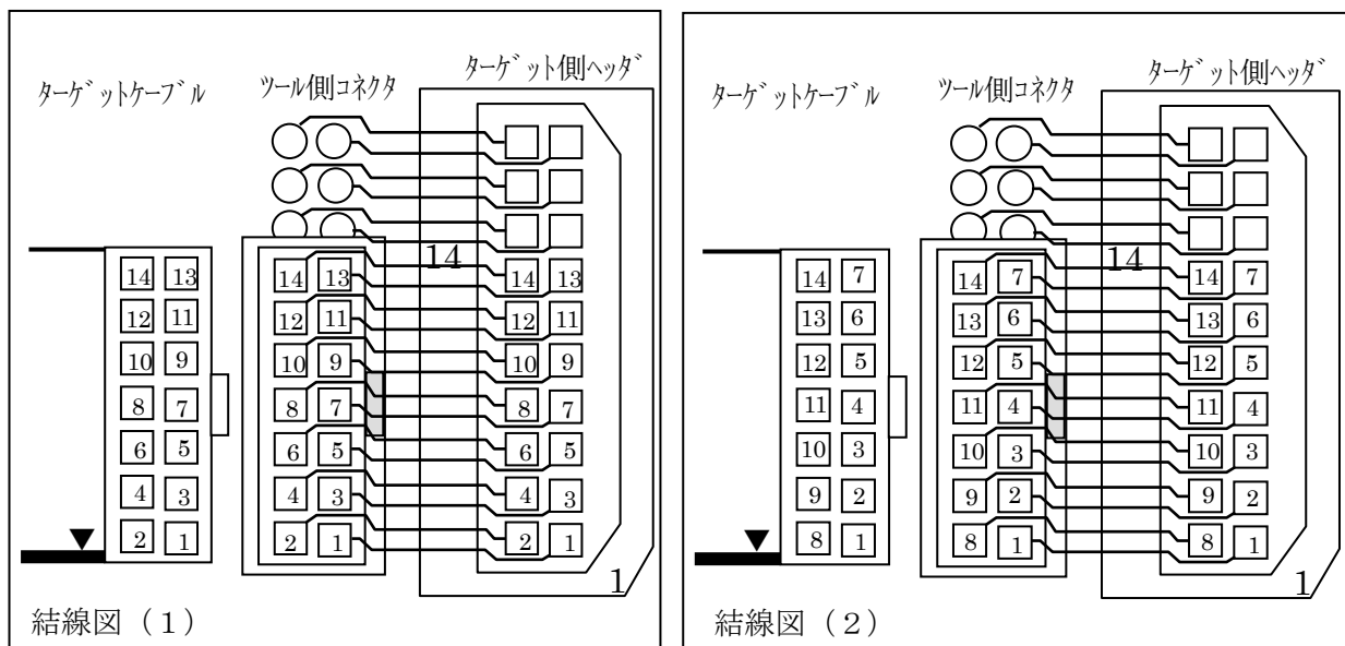
【図 4：結線情報】
