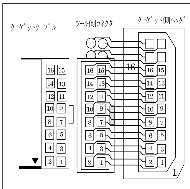
【図 4：結線情報】
