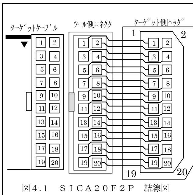
【図 4：結線情報】
