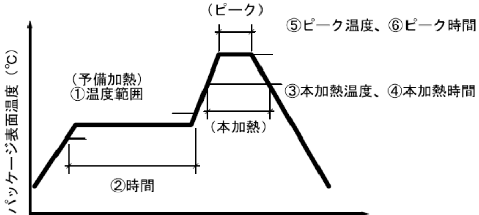
リフロー温度プロファイル
