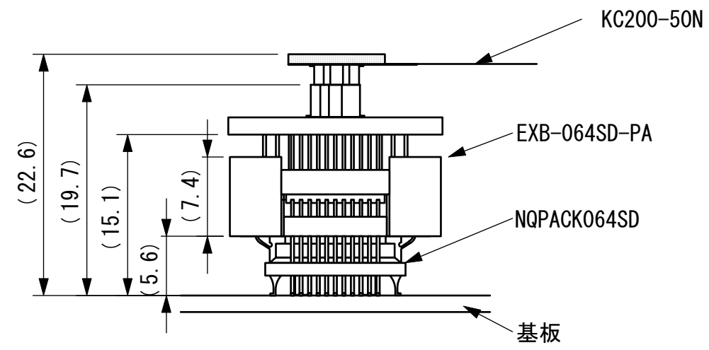
NQPACとの嵌合図 (2:1)
