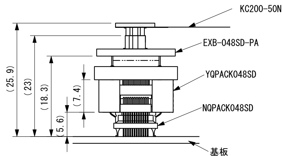
NQPACK、YQPACKとの嵌合図 (2:1)
