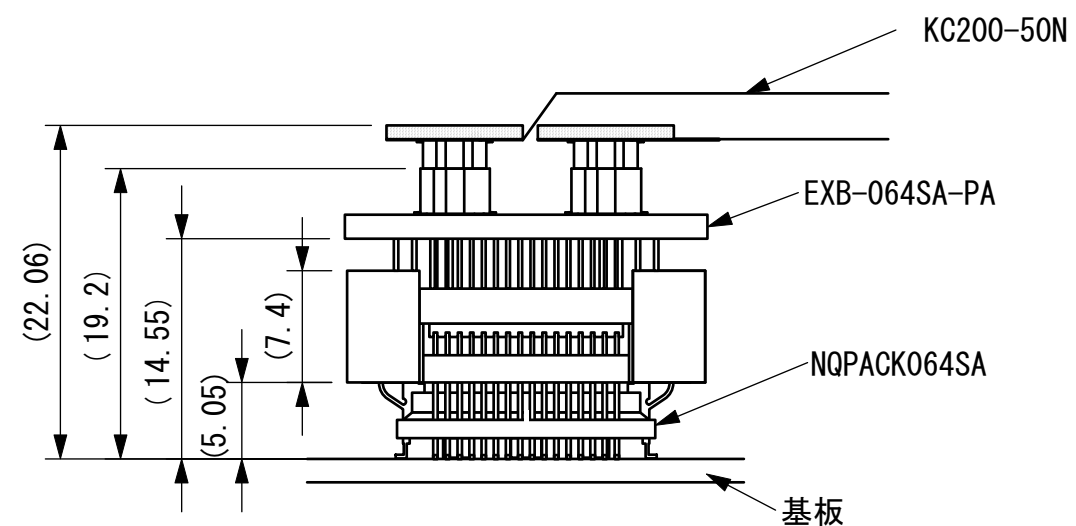
NQPACKとの嵌合図 (2 : 1)
