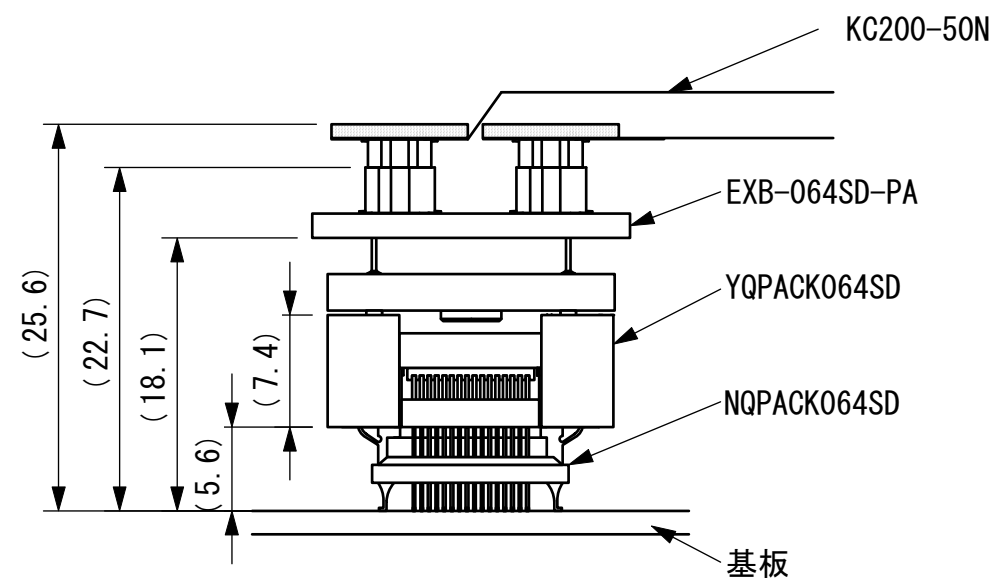
NQPACK、YQPACKとの嵌合図 (2 : 1)
