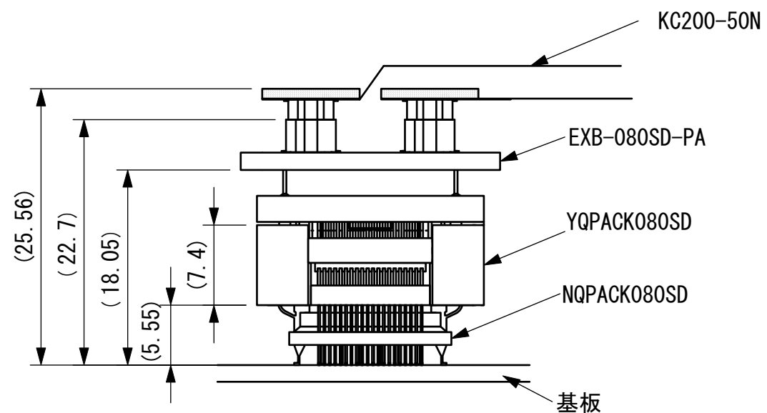
NQPACK、YQPACKとの嵌合図 (2 : 1)
