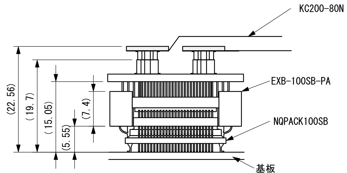
NQPACKとの嵌合図 (2 : 1)
