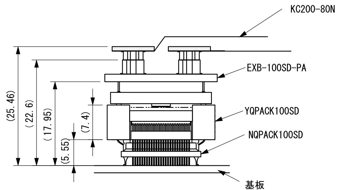
NQPACK、YQPACKとの嵌合図 (2:1)
