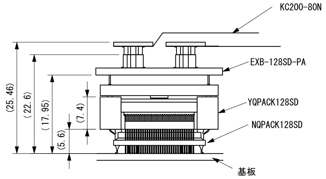
NQPACK、YQPACKとの嵌合図 (2 : 1)
