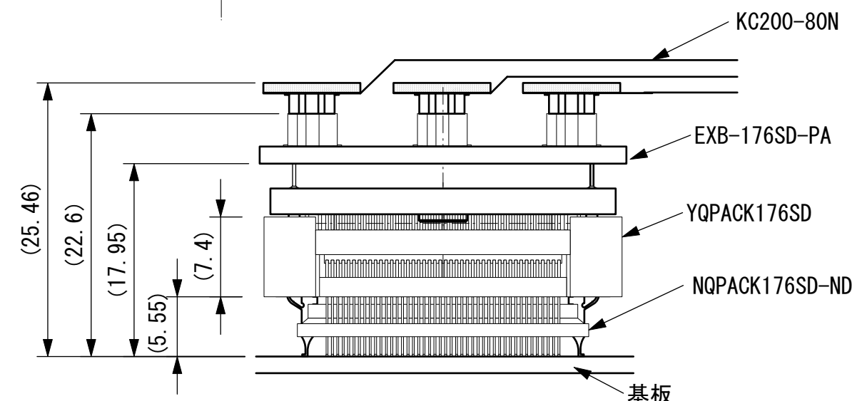
NQPACKとの嵌合図 (2 : 1)
