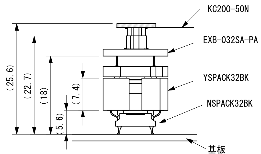
NSPACK、YSPACKとの嵌合図 (2:1)
